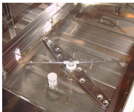
Površinski Inox filtri z Inox pomivalnimi in ločenimi Inox izpiralnimi rokami
